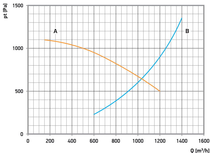
A - charakterystyka pracy N34 B - ramię DN 160 mm, L=3 m
